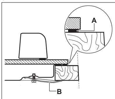
A) isporučena brtva B) isporučeni nosači
