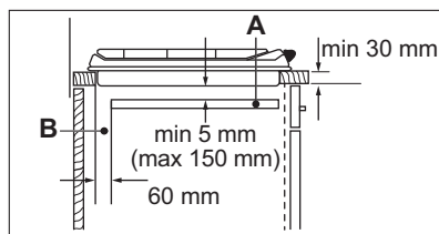
A. Ploča koja se može ukloniti B. Mjesto za priključke
