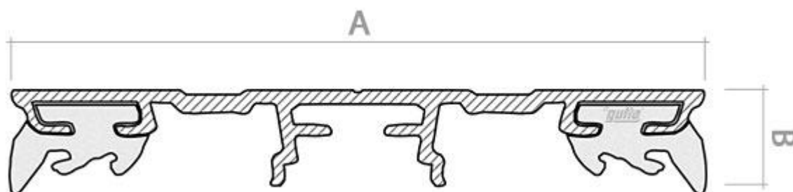
Skica: Spojni profil Guttaprofil ALU univerzalni s brtvama
