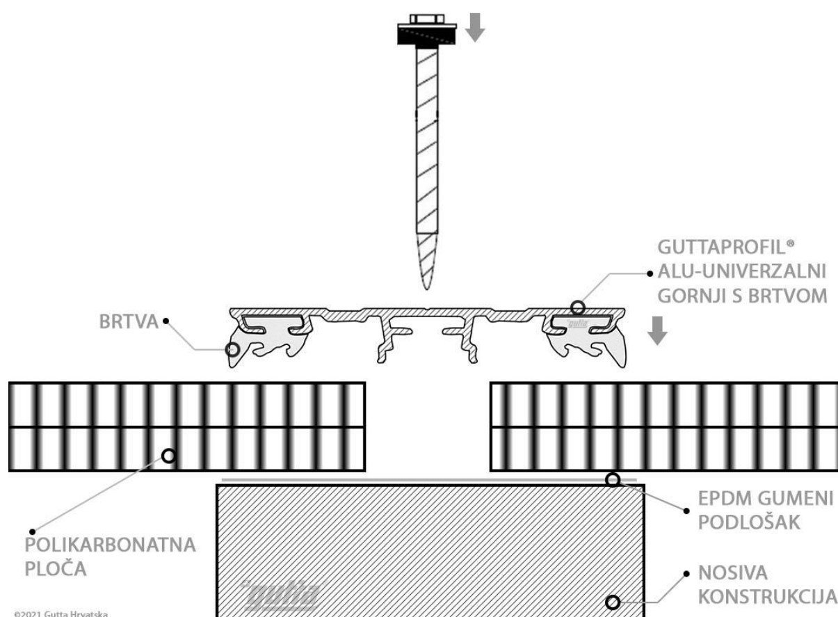
Skica: pričvršćivanje višeslojnih ili kompaktnih ploča od polikarbonata ili akrila na potkonstrukciju uz upotrebu univerzalnog vijka i spojnog Guttaprofila
